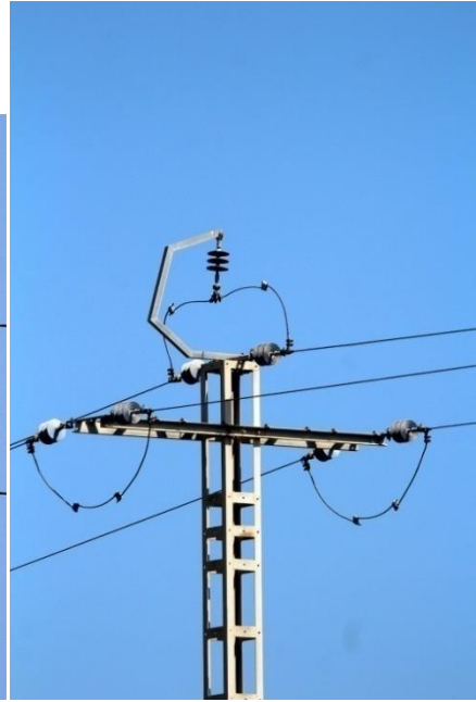
Crucetas en cruz. Aisladores rígido (hacia arriba) y en cadena (horizontales). Cadena de amarre.
