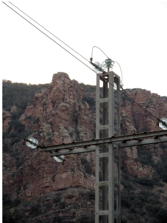
Cruceta en cruz. Aislador rígido (arriba), y en cadena de amarre.
