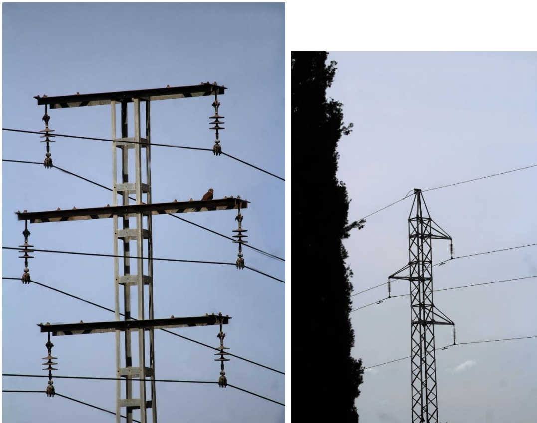
Cruceta a tresbolillos. Aisladores suspendidos
