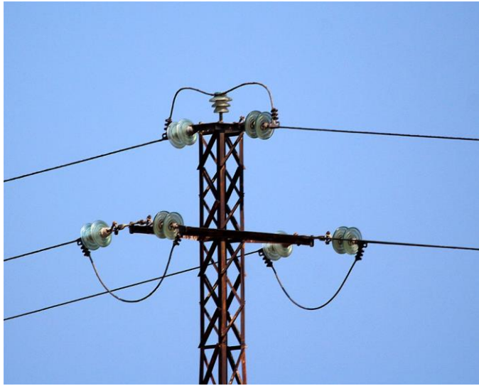
Crucetas en cruz. Aisladores rígido (hacia arriba) y en cadena (horizontales). Cadena de amarre.
