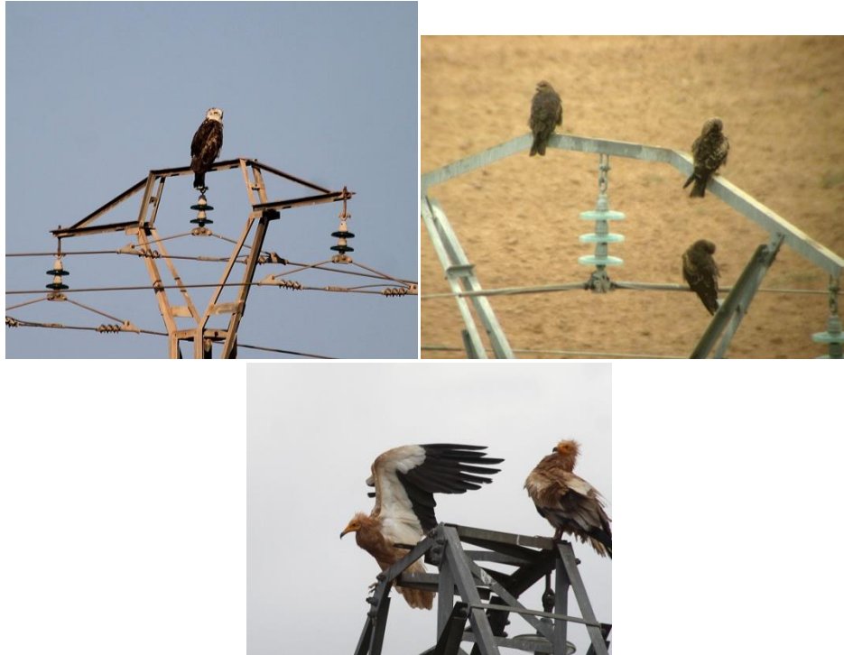
Crucetas de bóveda con aisladores suspendidos.
